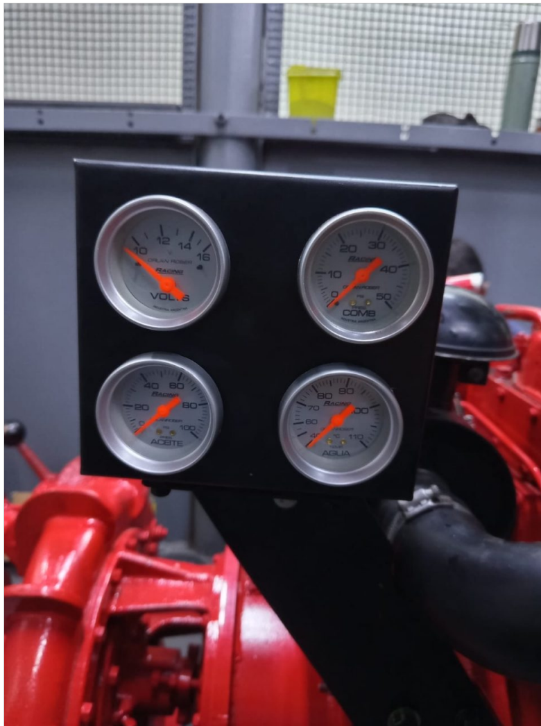
Moto-Bomba (Perkins 4-203) - Instalacion de pirometria.
