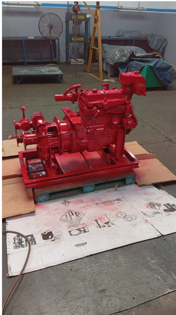
Moto-Bomba (Perkins 4-203) - Alistamiento para traslado.
