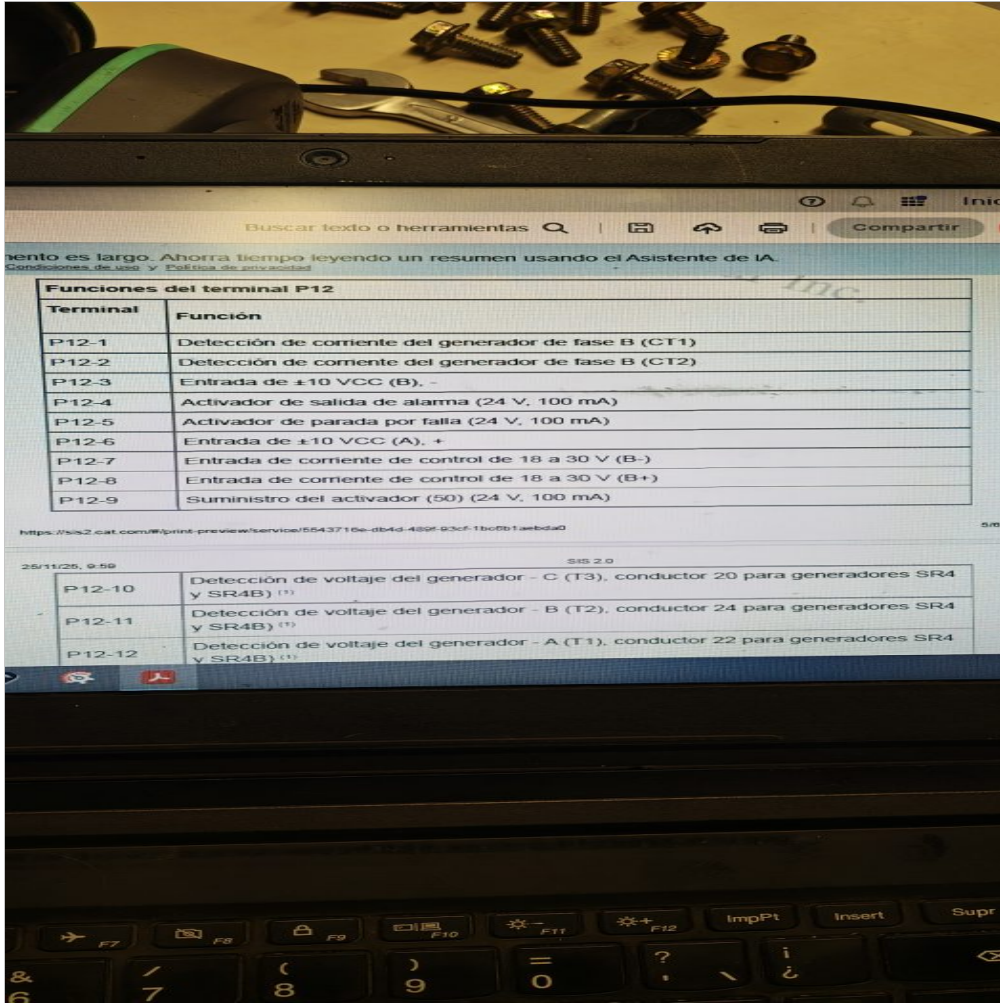
Funciones de la ficha P-12
